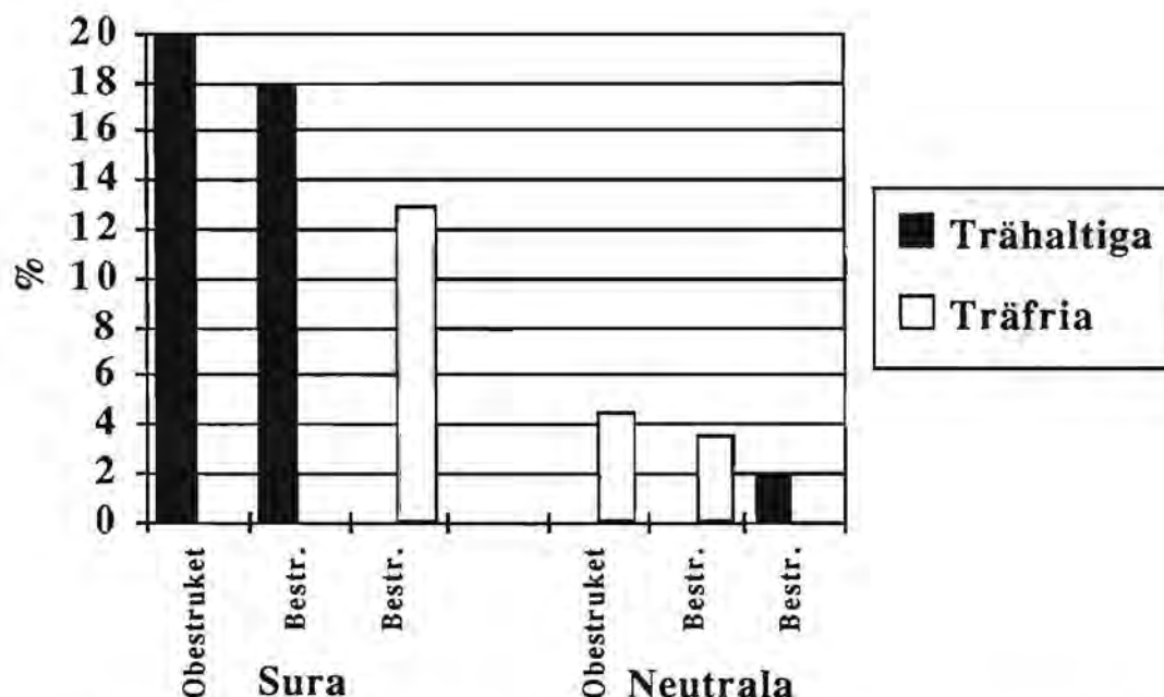
Figur. Åldringsbeständighet hos obestrukna och bestrukna pappersark mätt som minskad rivstyrka i procent efter accelererad åldring i 80 °C/65 % rel. fuktighet. Neutrala papper har den bästa hållbarheten.
