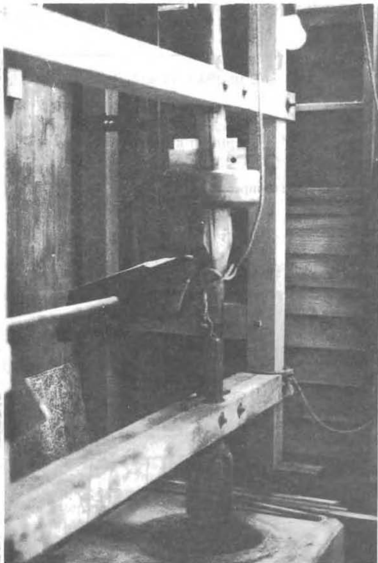
Stamparna lyfts av kamaxeln.
