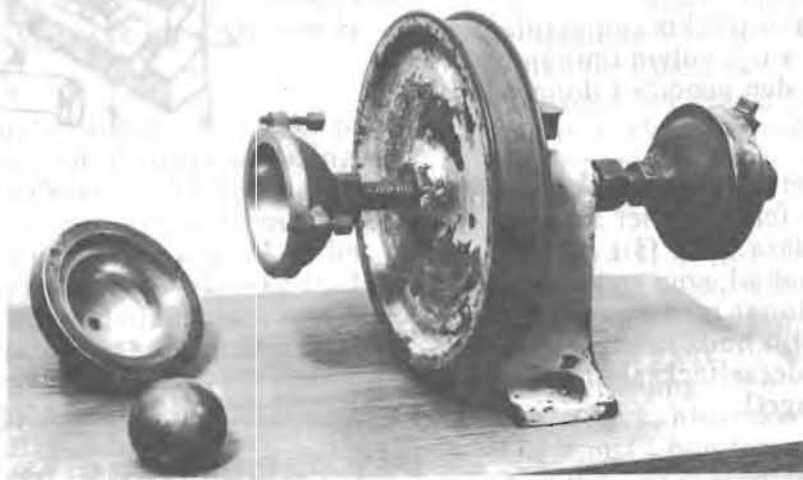
En Lampén-kvarn i originalversion från Centrallaboratoriets tidiga års metodforskning. Denna utvecklades sedan till en standardkvarn som användes i laboratorier på olika håll i världen
